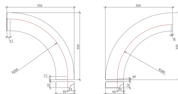
ЧЕРТЁЖ РАДИУСНЫХ БАГЕТОВ
