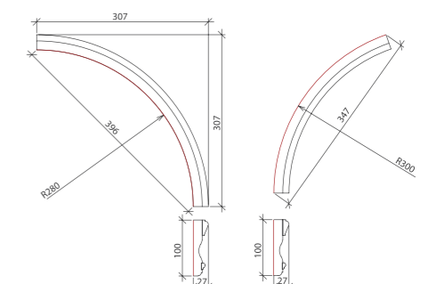
ЧЕРТЁЖ РАДИУСНЫХ БАГЕТОВ
