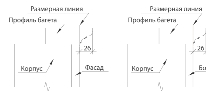
РАСПОЛОЖЕНИЕ БАГЕТОВ НА КОРПУСЕ
