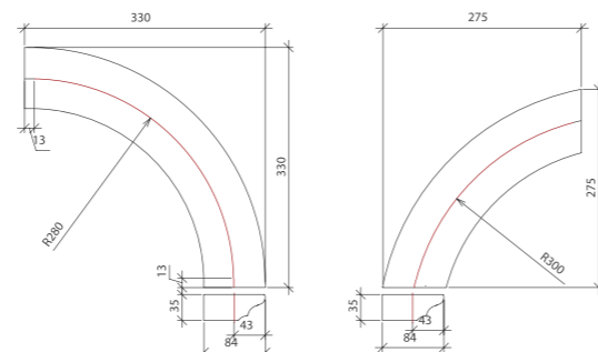
ЧЕРТЁЖ РАДИУСНЫХ БАГЕТОВ
