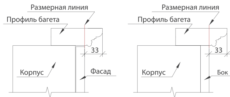
РАСПОЛОЖЕНИЕ БАГЕТОВ НА КОРПУСЕ
