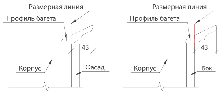
РАСПОЛОЖЕНИЕ БАГЕТОВ НА КОРПУСЕ
