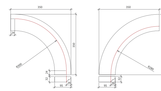
ЧЕРТЁЖ РАДИУСНЫХ БАГЕТОВ
