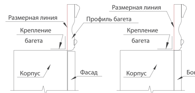
РАСПОЛОЖЕНИЕ БАГЕТОВ НА КОРПУСЕ
