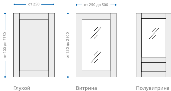
Глухой
